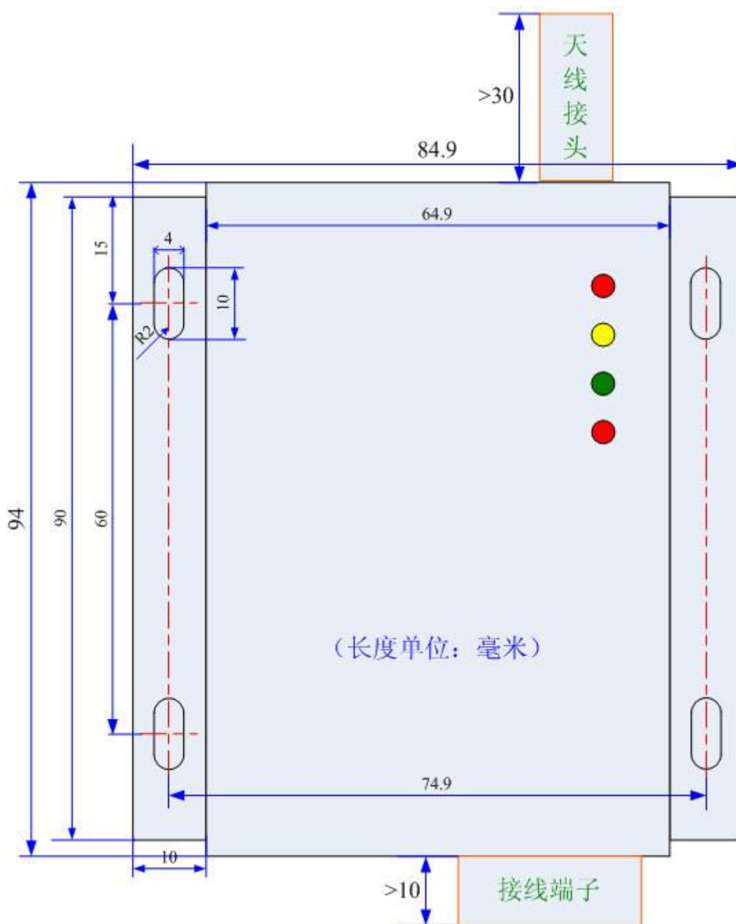
产品外形尺寸图
