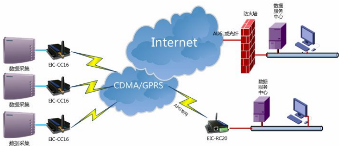
（图一） DTU远程监控系统
