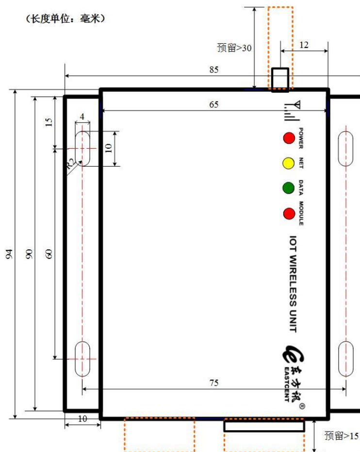
(图3) 产品外形尺寸图
