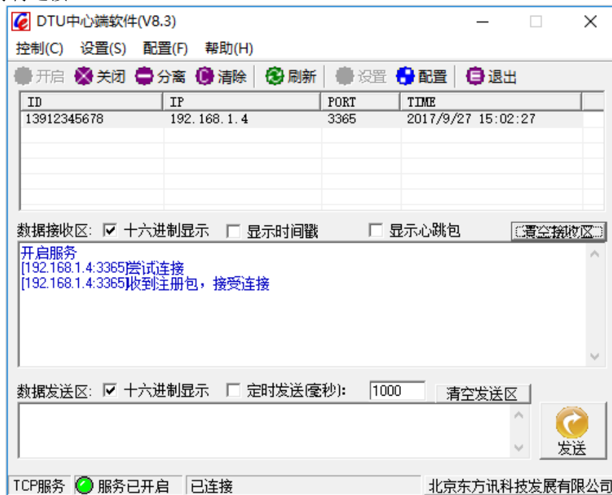
(图13) DTU中心端软件
