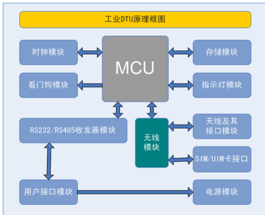
(图2) DTU原理框图
