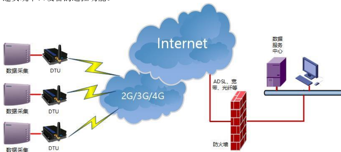
（图1） DTU远程监控系统
