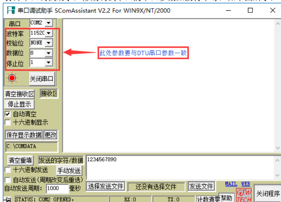
(图14) 串口调试助手配置
