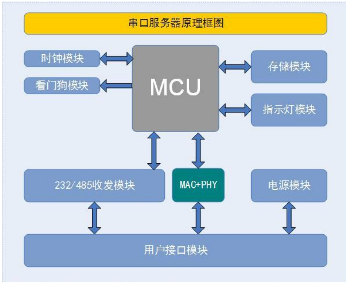
(图2) 串口服务器原理框图
