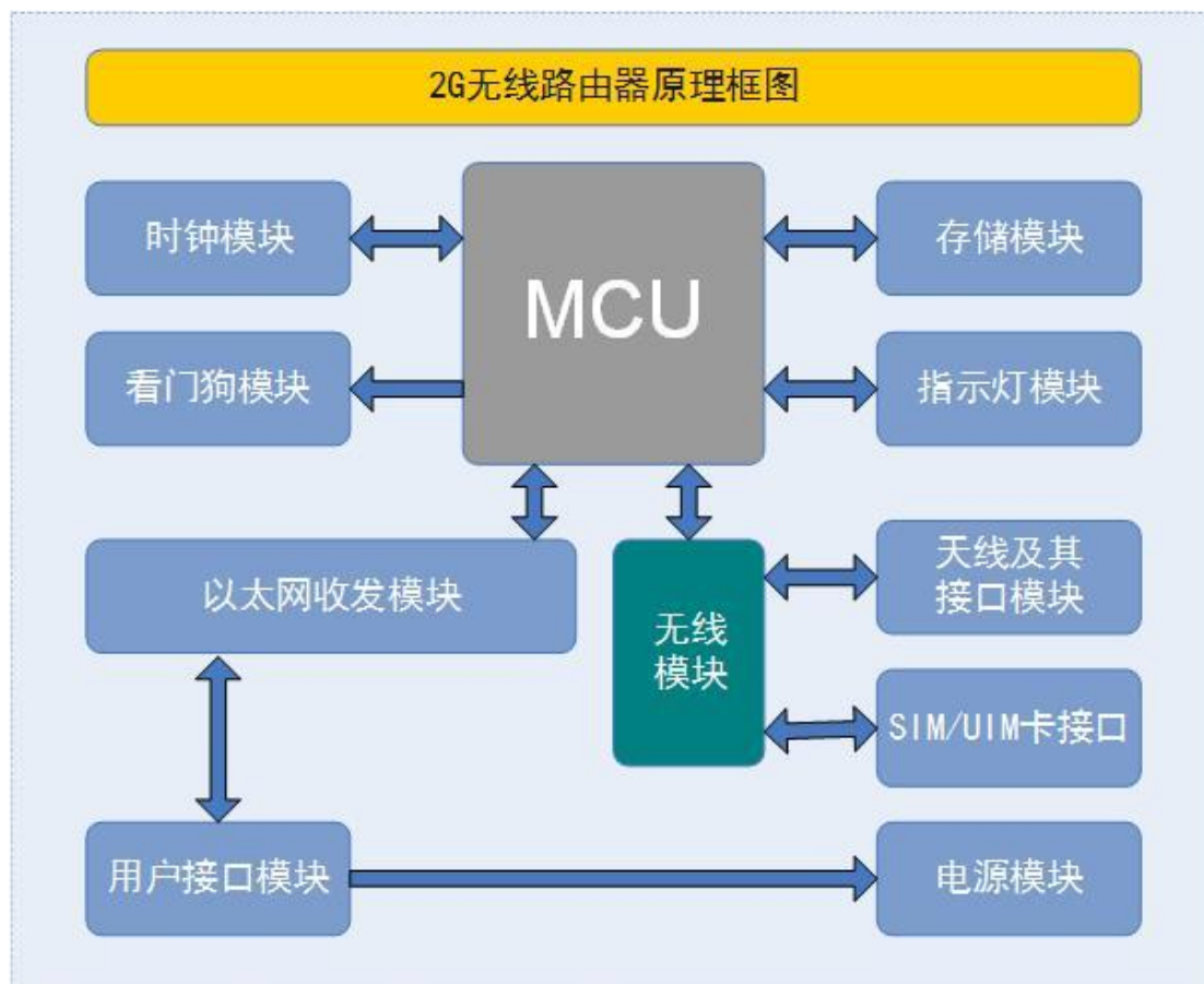
(图2) CDMA无线路由器原理框图
